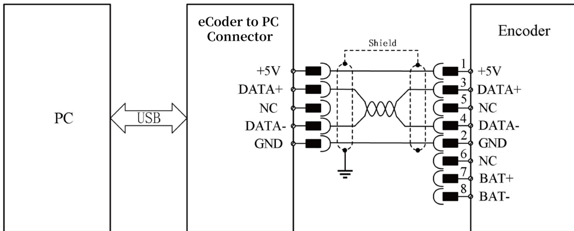
图 10-2 接线示例图
