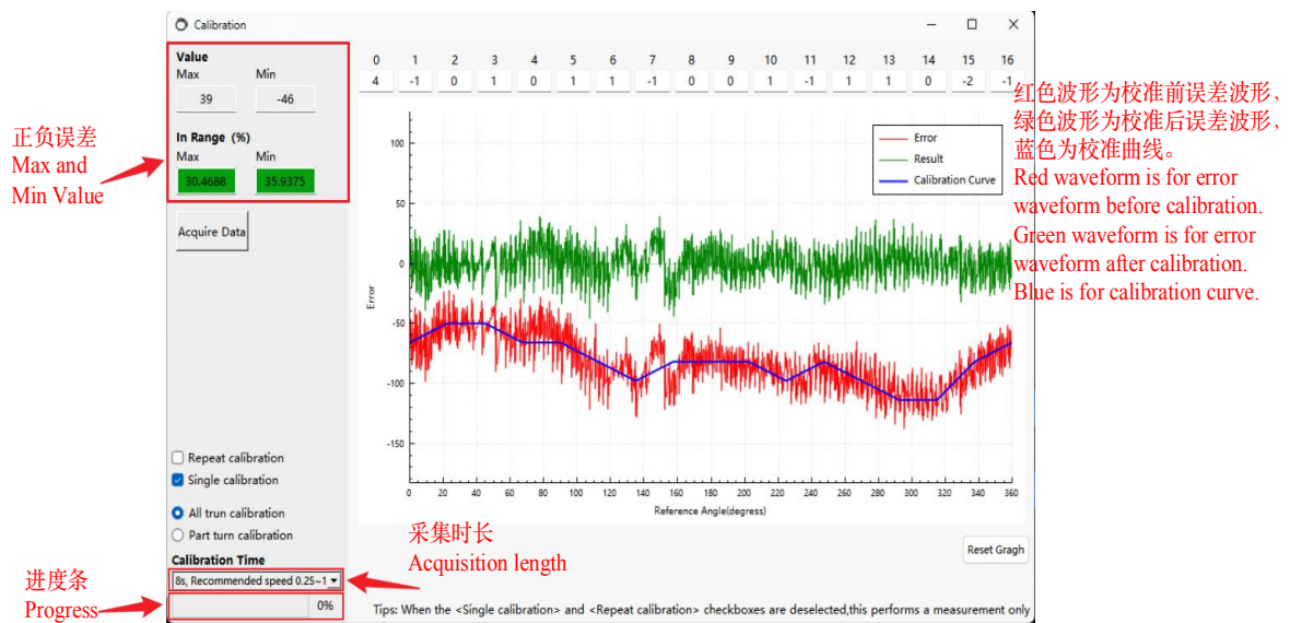
图 11-4 编码器校准与测量
