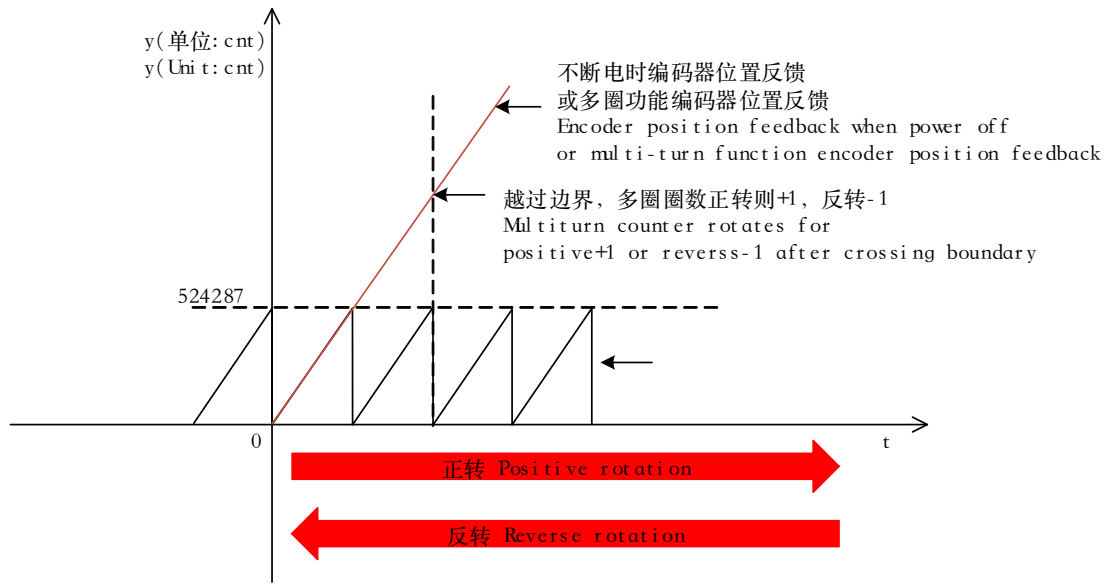
图 9-1 位置反馈
