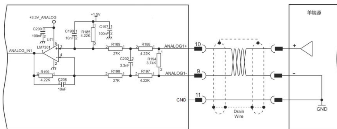
差分模拟输入 – 推荐连接图
