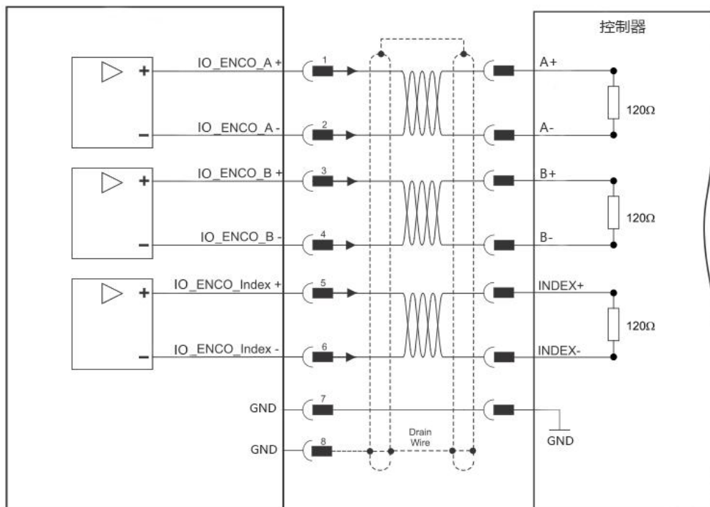
编码器差分信号输出 – 推荐连接图
