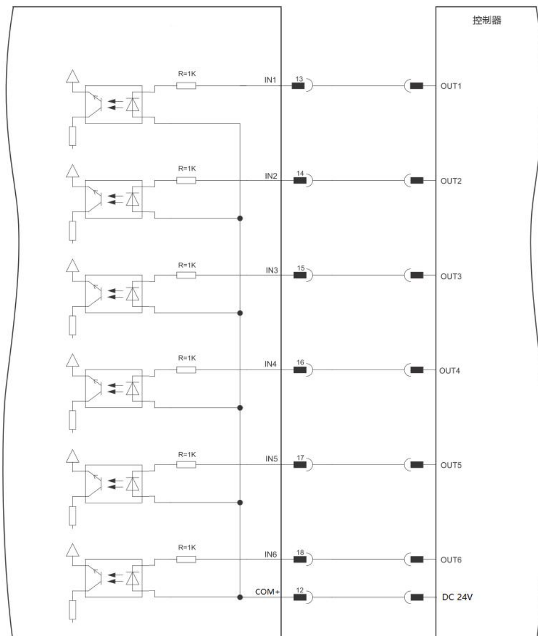
数字输入 – 推荐连接图
