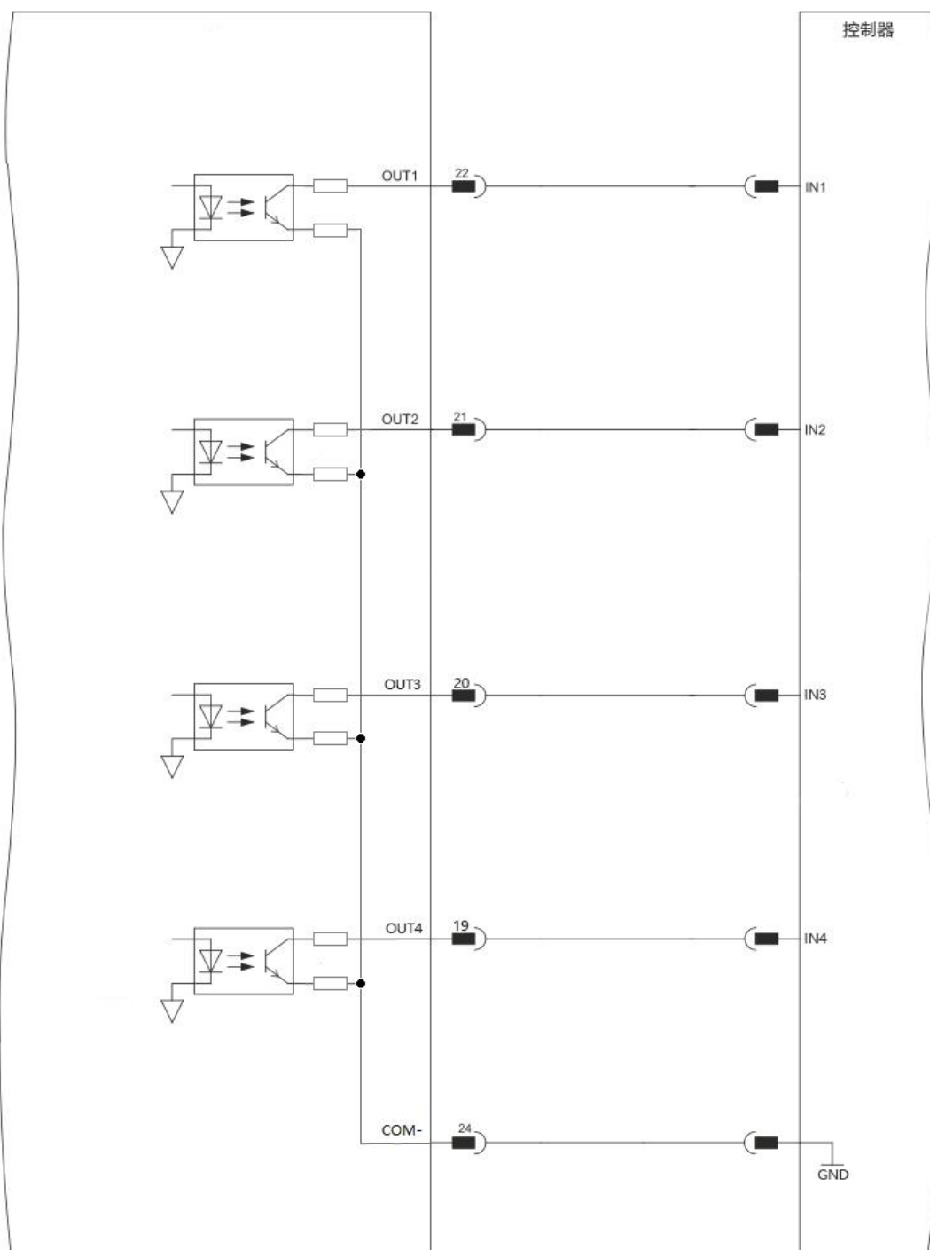
数字输出 - 推荐连接图
